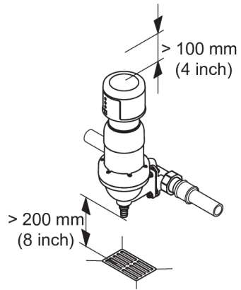
JPF+-A 1½" - 2"
