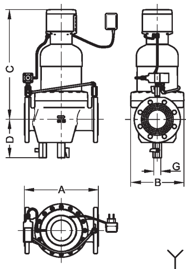
Fig. 11: JPF-A DN 65 - 100
