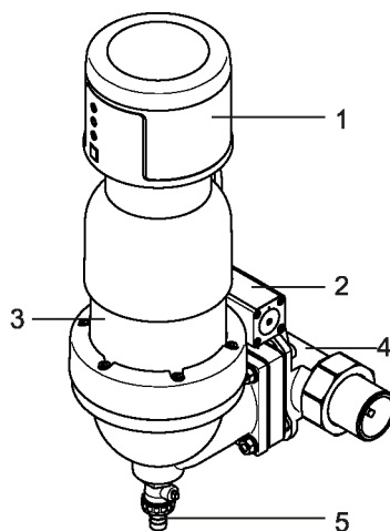
Fig. 2: JPF+-A 1½" - 2"
